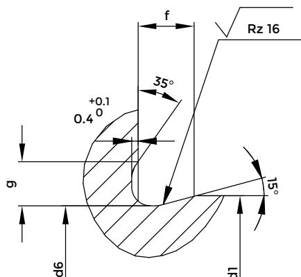
Dettaglio Y
