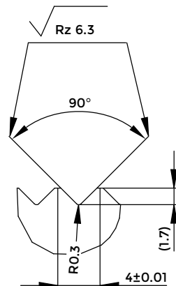
Dettaglio Z
