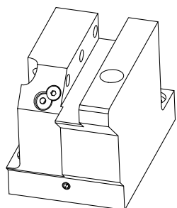
137-00297 (sinistro) 20x20 mm
