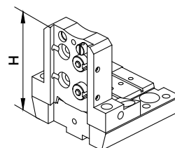
121-22076 (h=32 mm - H=100 mm)
